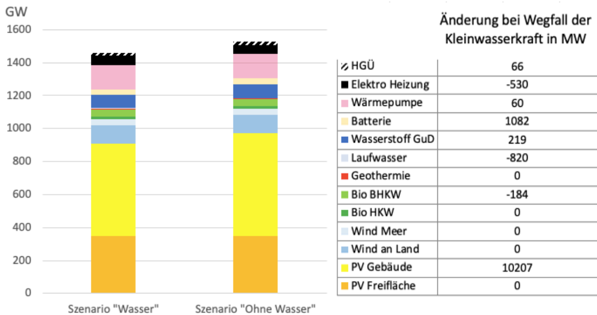
Abbildung 1: Optimisiertes Energiesystem für alle Energiesektoren in Deutschland in den Szenarien Wasser und Ohne Wasser (Grafik), und entsprechend notwendige Änderung des Energiesystems bei Wegfall der Kleinwasserkraftwerke bis 1000 kW (Tabelle).
